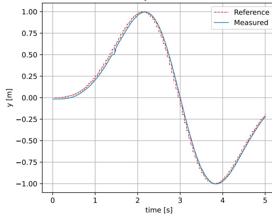
y State
